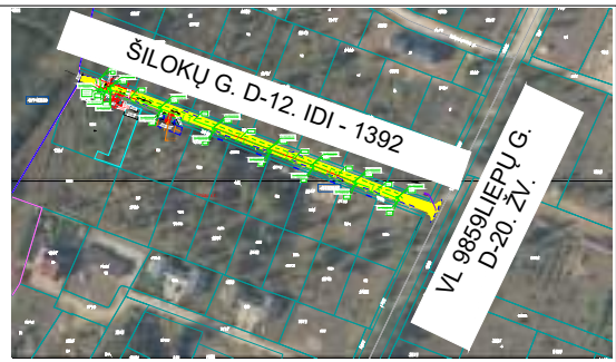
SITUACIJOS PLANAS
