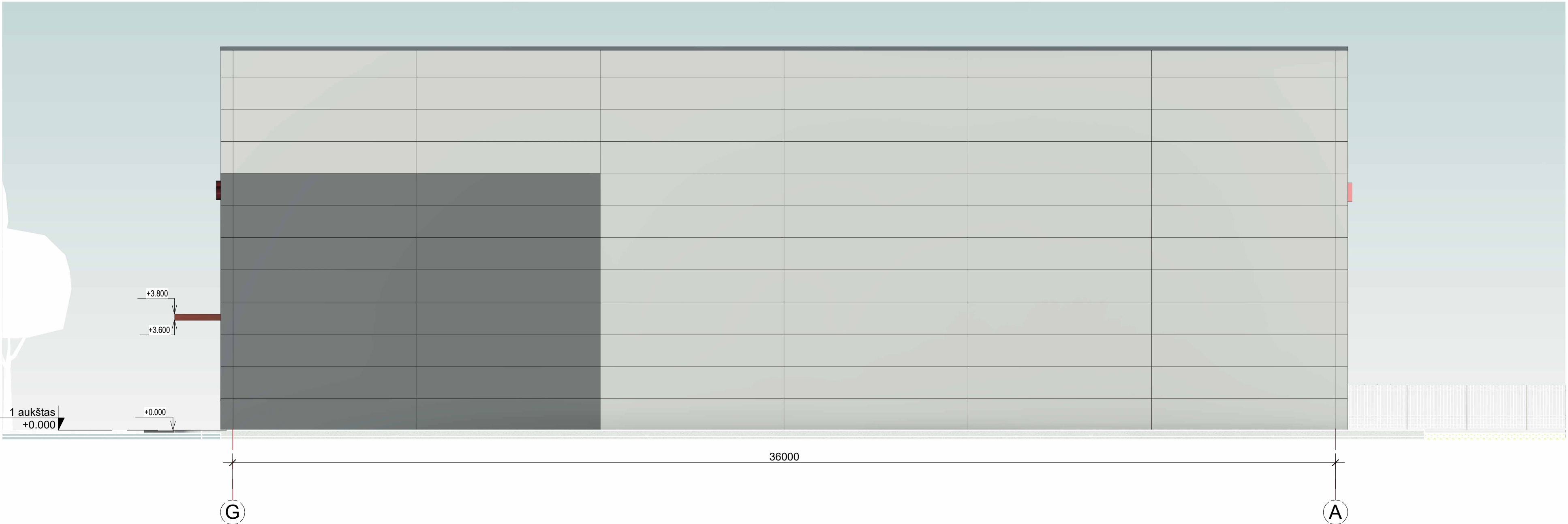
2 Rytu fasadas. Apdaila 1 : 100
