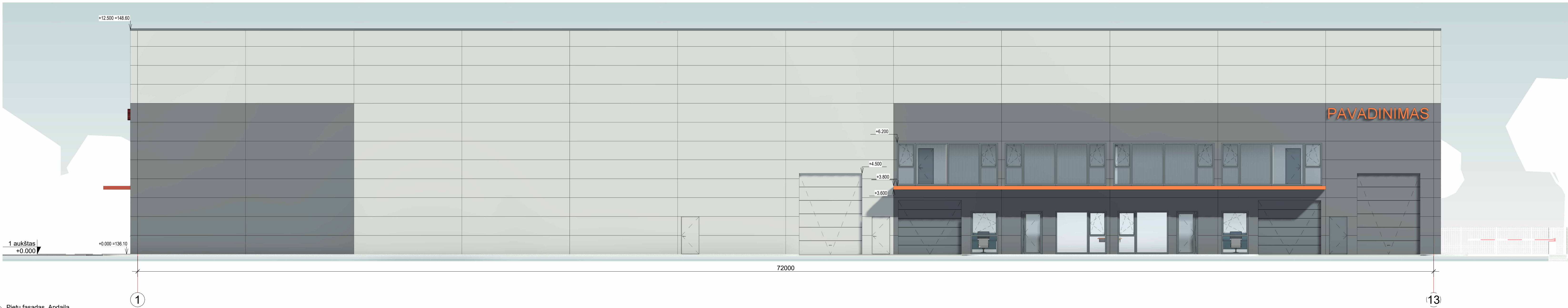
3 Pietu fasadas. Apdaila 1 : 100
