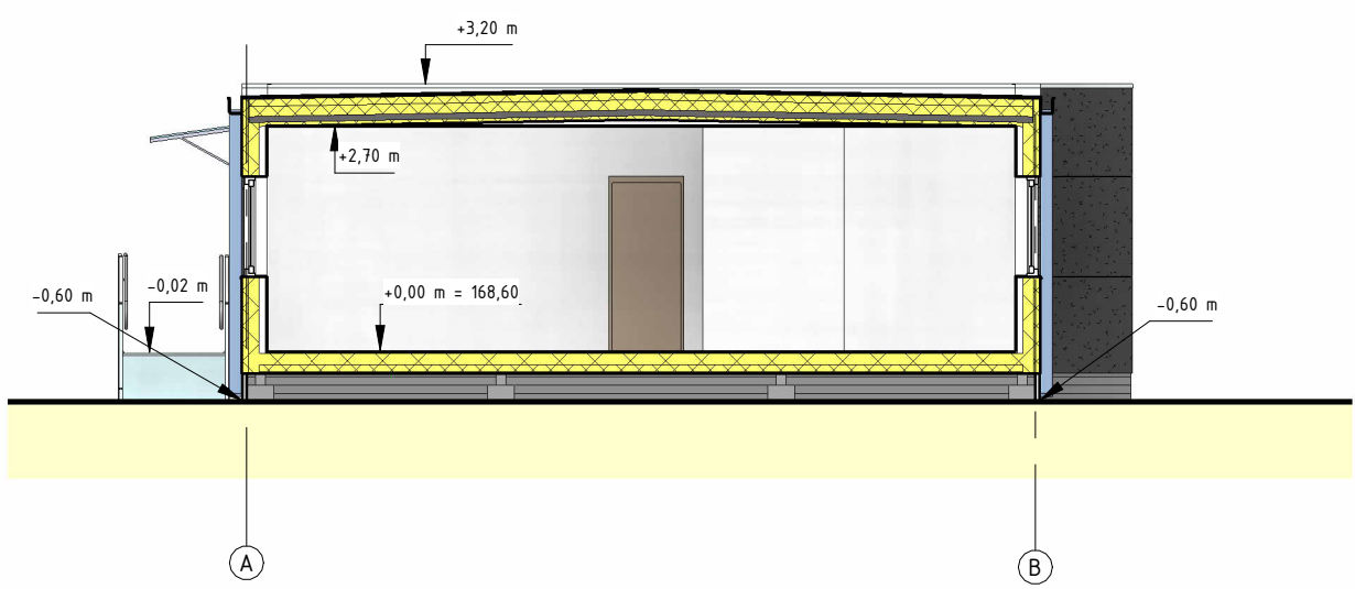
PJŪVIS 1-1 1 : 100
