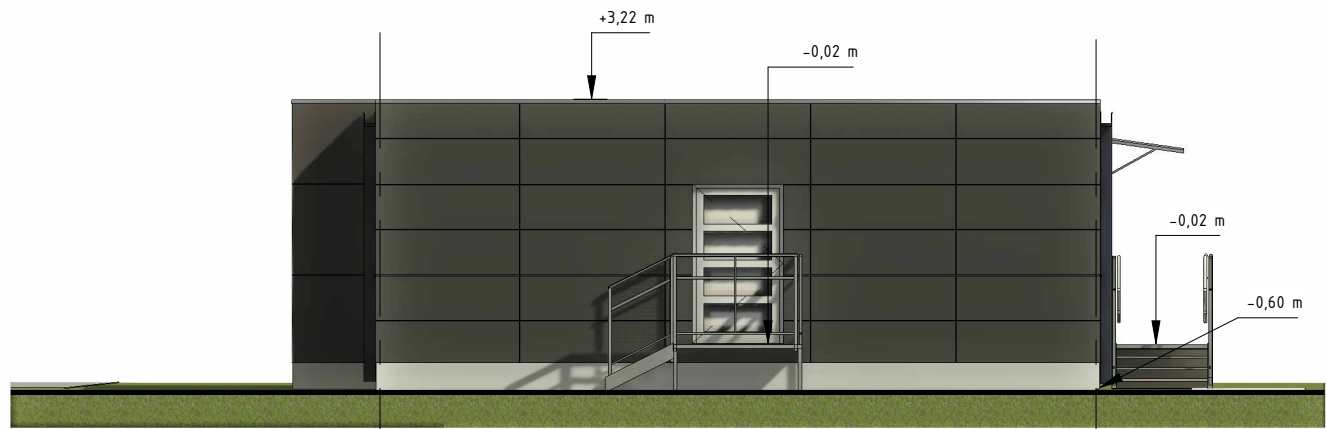
FASADAS B-A 1 : 100
