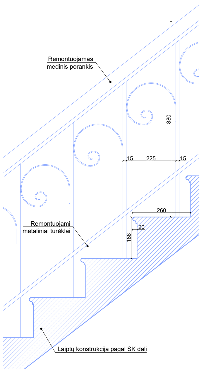
TURĖKLŲ T_2 DETALĖ. M1:10
