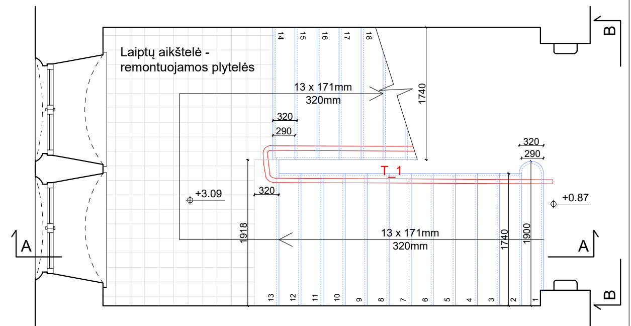
LAIPTŲ LP_1 PIRMO AUKŠTO PLANAS. M1:50
