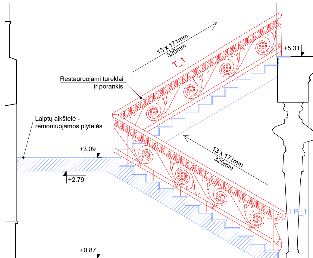
PJŪVIS A-A. M1:50
