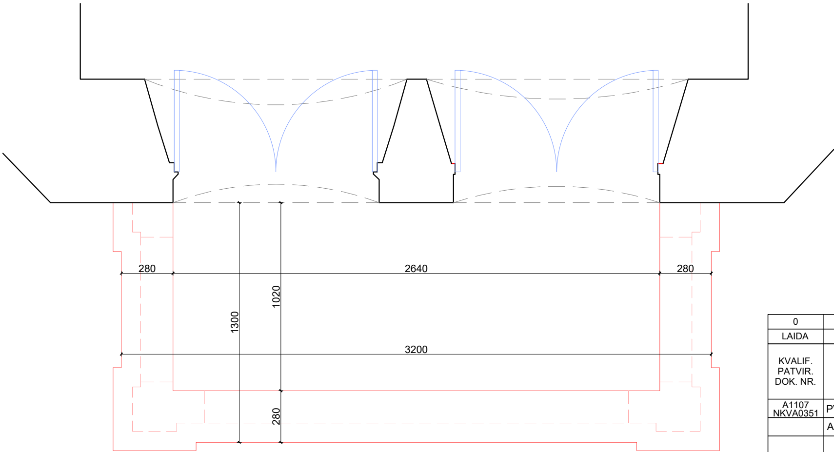
ATKURIAMO BALKONO PLANAS. M1:20
