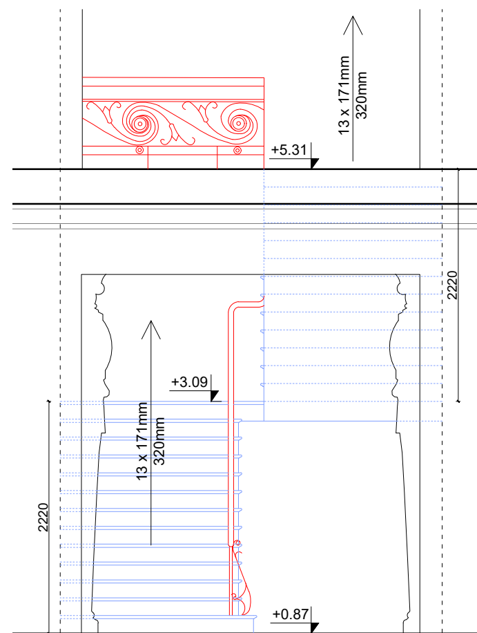
PJŪVIS B-B. M1:50
