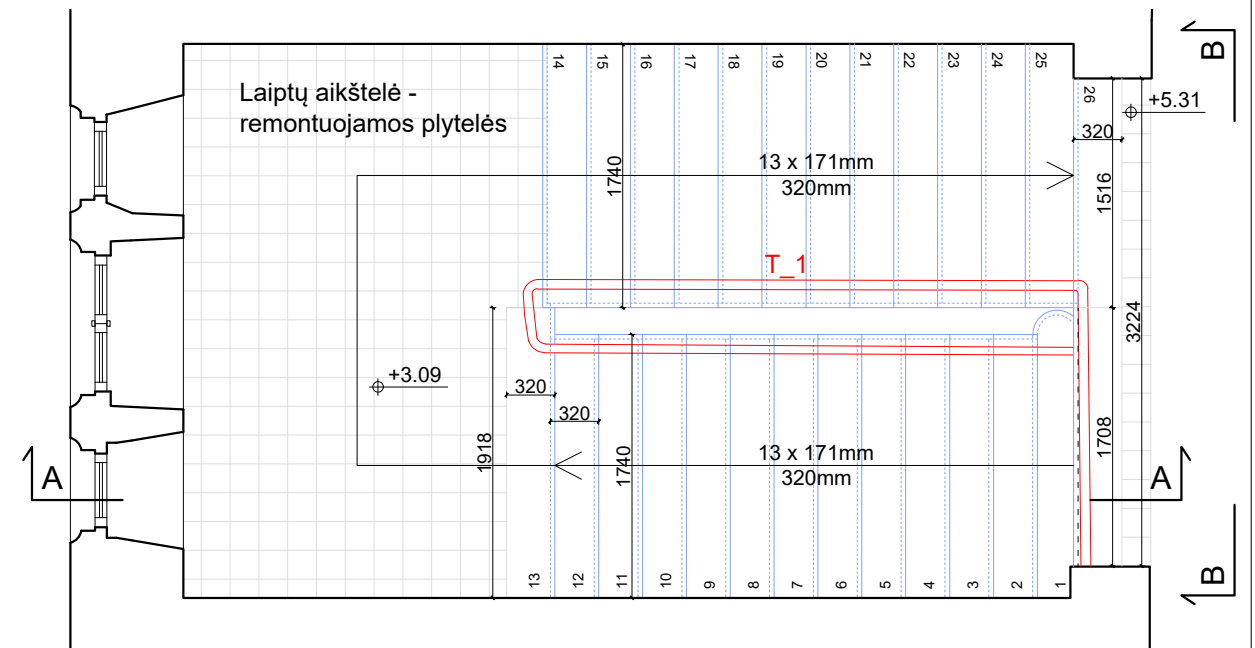
LAIPTŲ LP_1 ANTRO AUKŠTO PLANAS. M1:50
