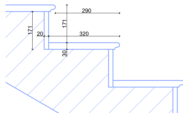
LAIPTŲ LP_1 DETALĖ. M1:10
