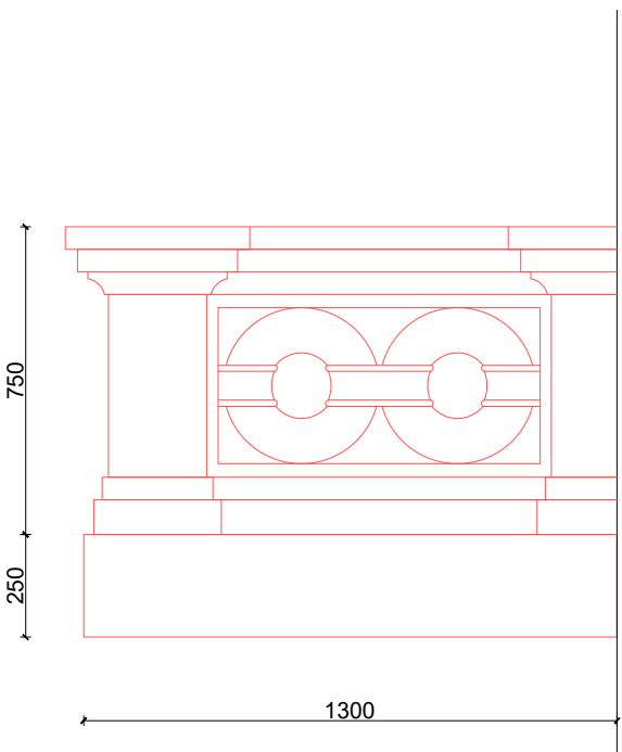
ATKURIAMO BALKONO VAIZDAS IŠ ŠONO. M1:20
