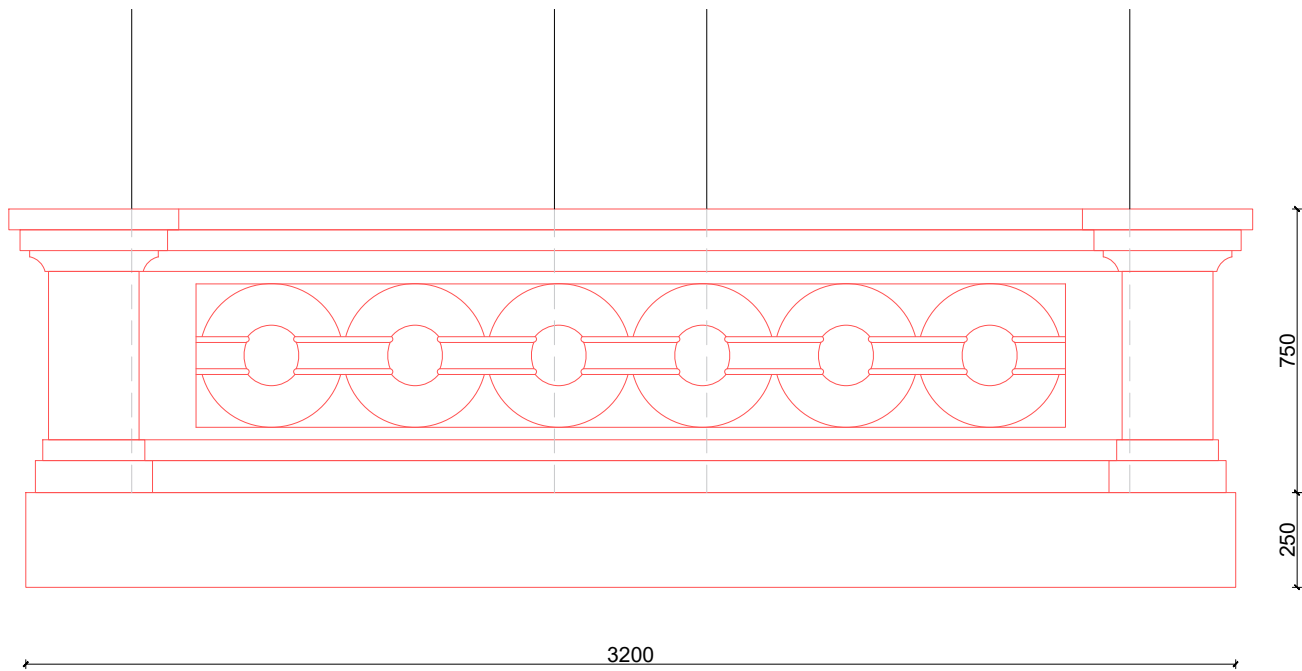
ATKURIAMO BALKONO VAIZDAS IŠ PRIEKIO. M1:20
