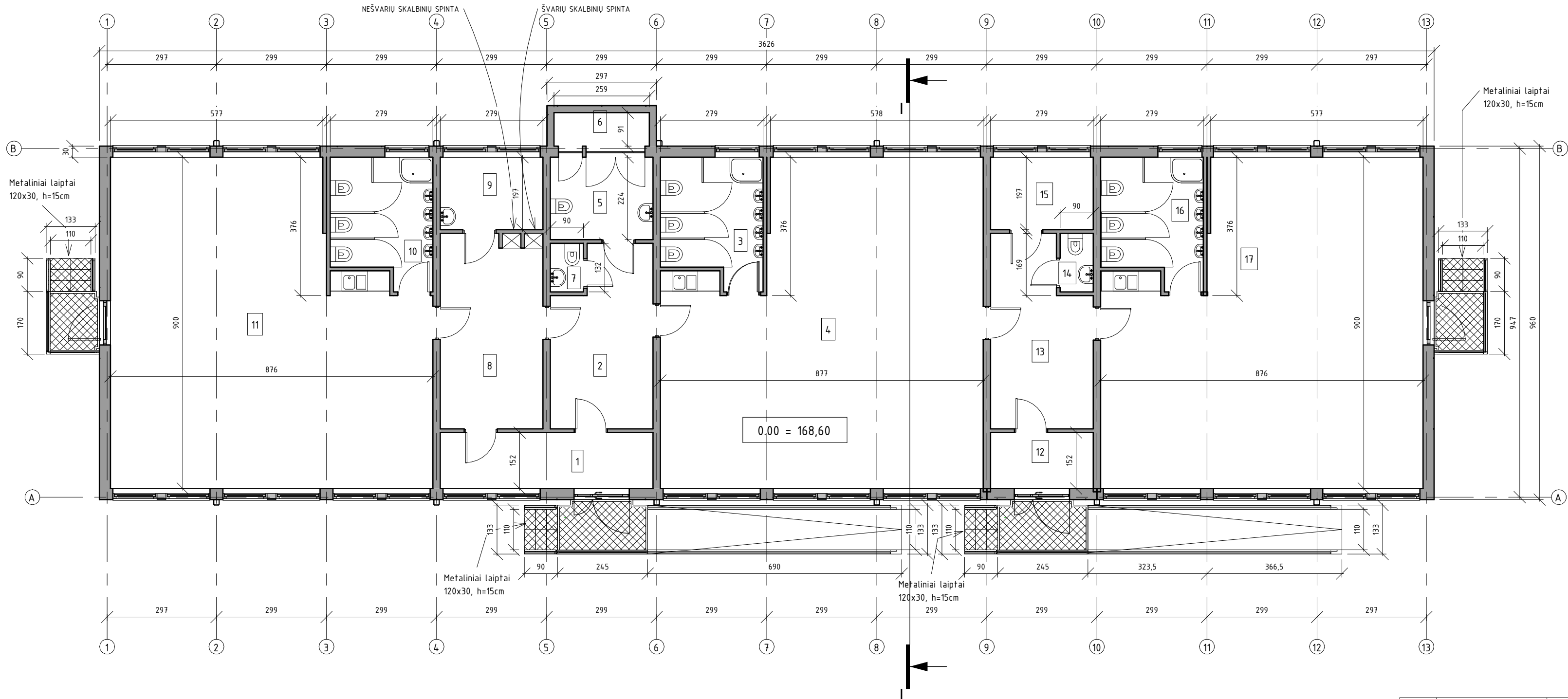
PLANAS 1 : 100
