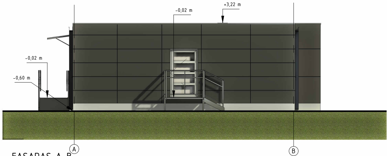
FASADAS A-B 1 : 100
