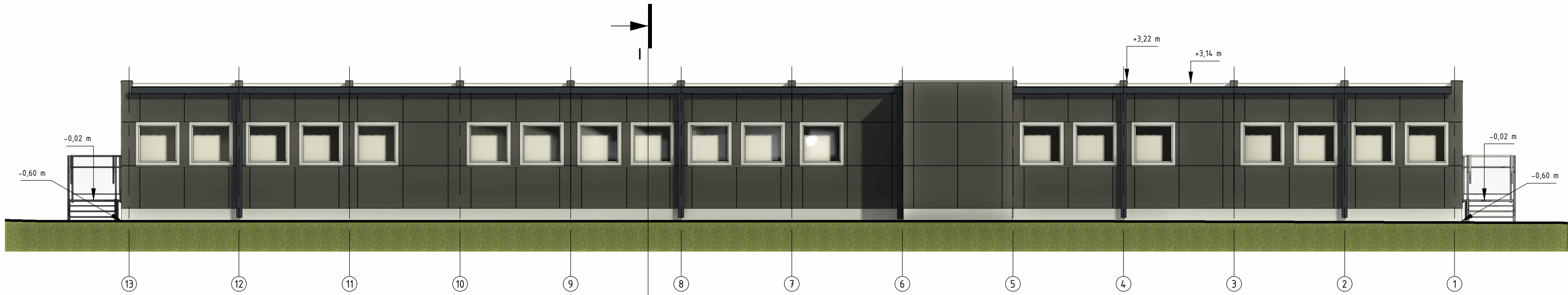
FASADAS 13-1 1 : 100
