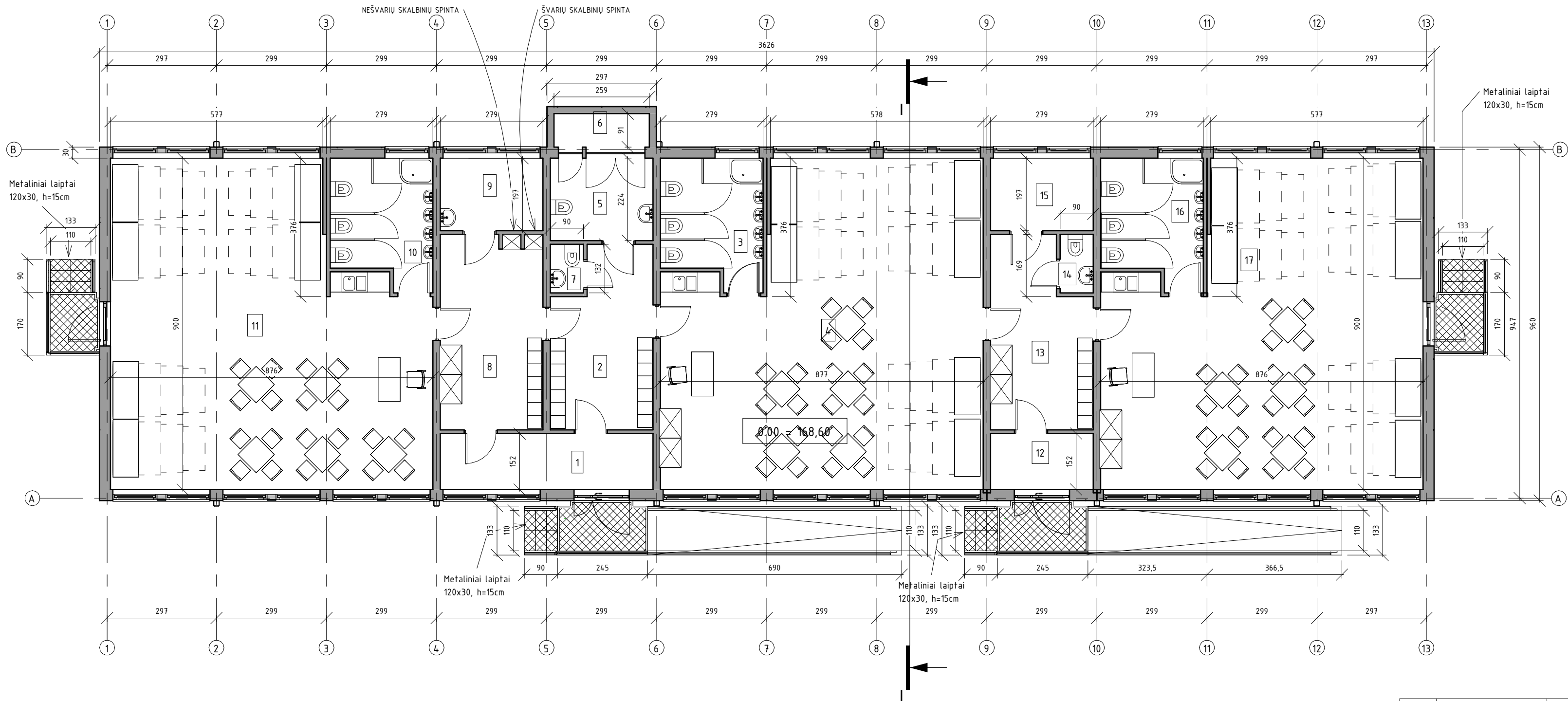
PLANAS 1 : 100
