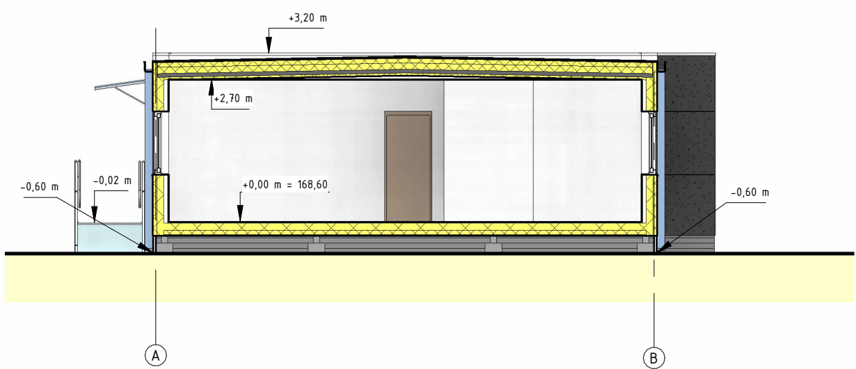
PJŪVIS 1-1 1 : 100
