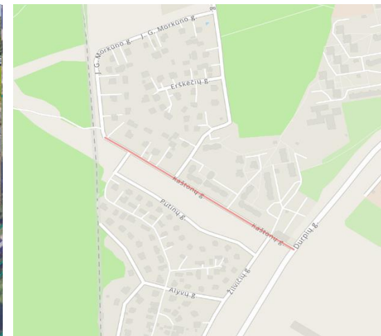
Situacijos schema.
