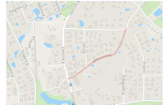
Situacijos schema.
