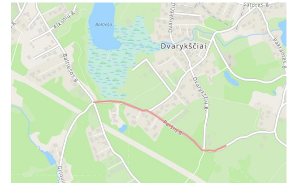
Situacijos schema.
