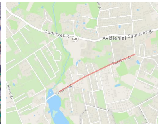
Situacijos schema
