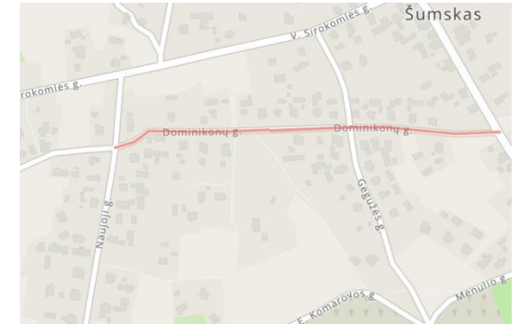
Situacijos schema.
