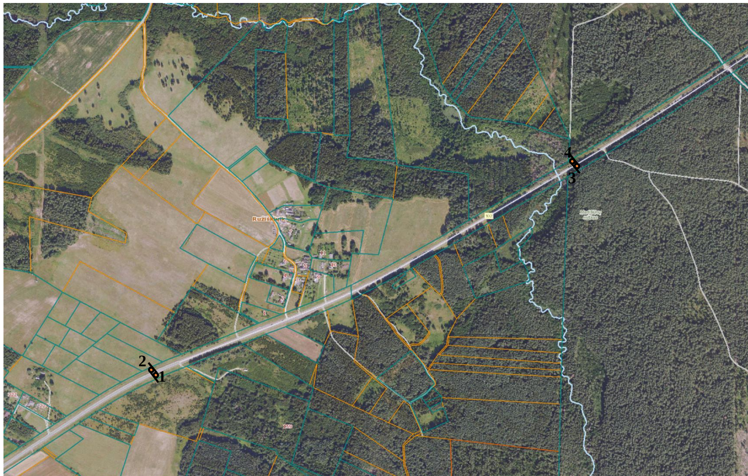
Situacijos schema
