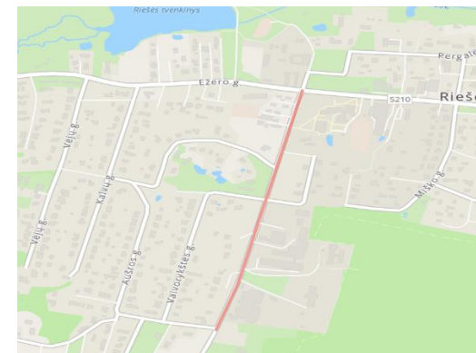
Situacijos schema.
