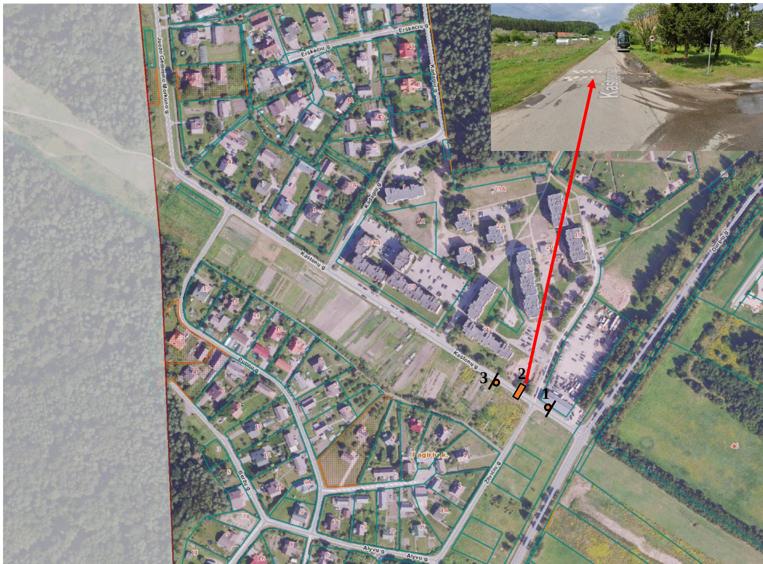
Situacijos schema.
