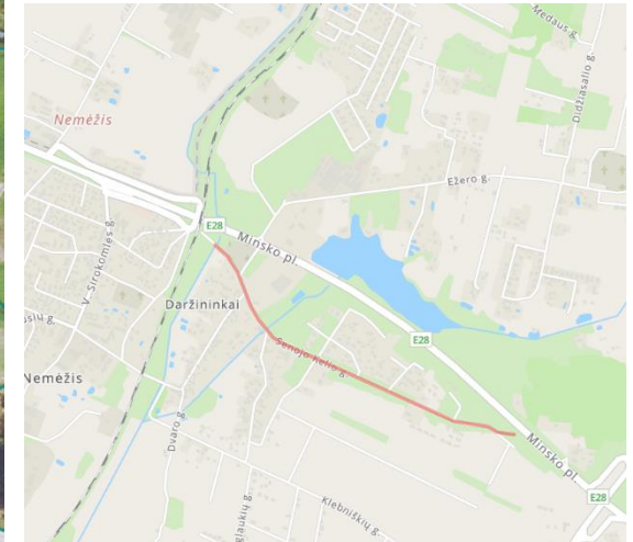
Situacijos schema.
