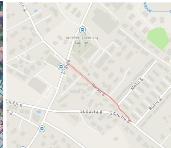
Situacijos schema.
