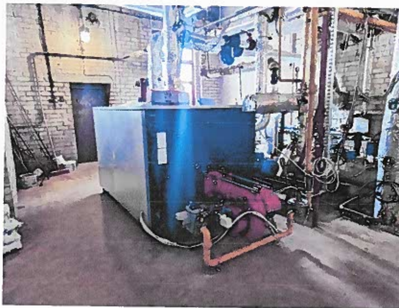
Katilas Unical TRISTAR 1400 2 S, Kranto 24 katilinėje
